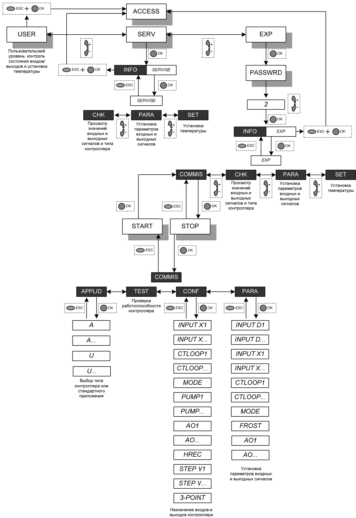
Рисунок 8. Схема программирования контроллеров.
