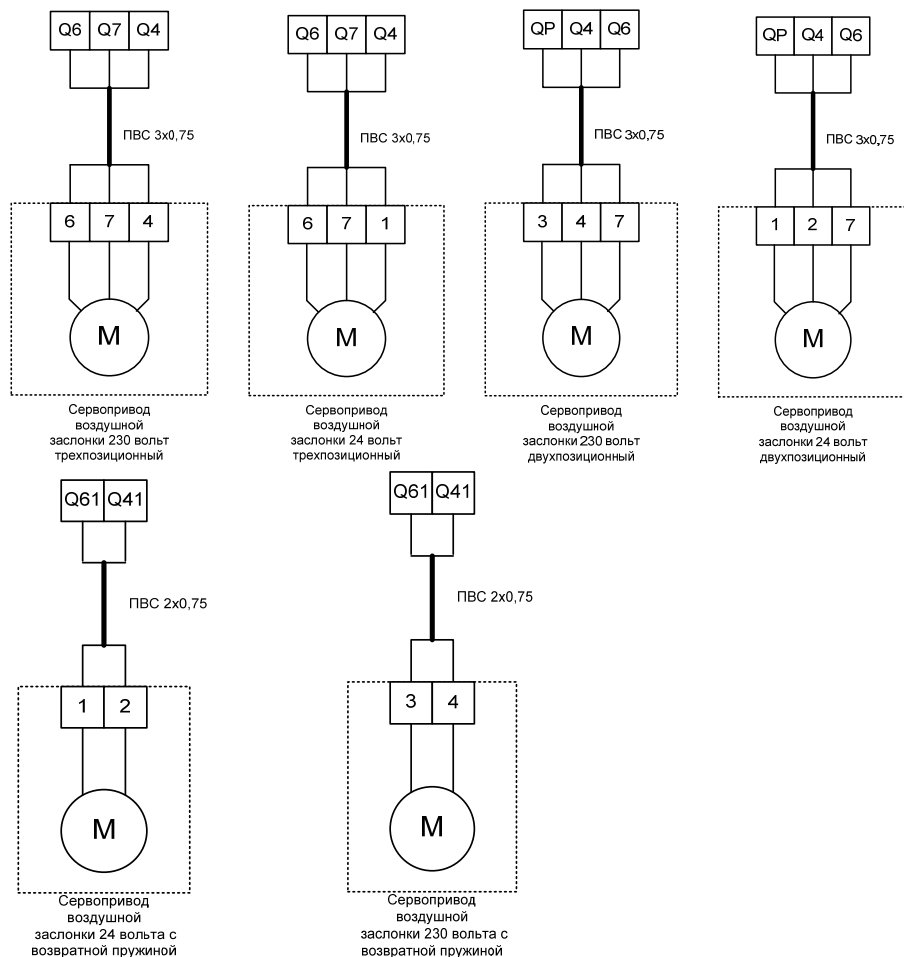
Рисунок 5. Подключение заслонок наружного воздуха.
