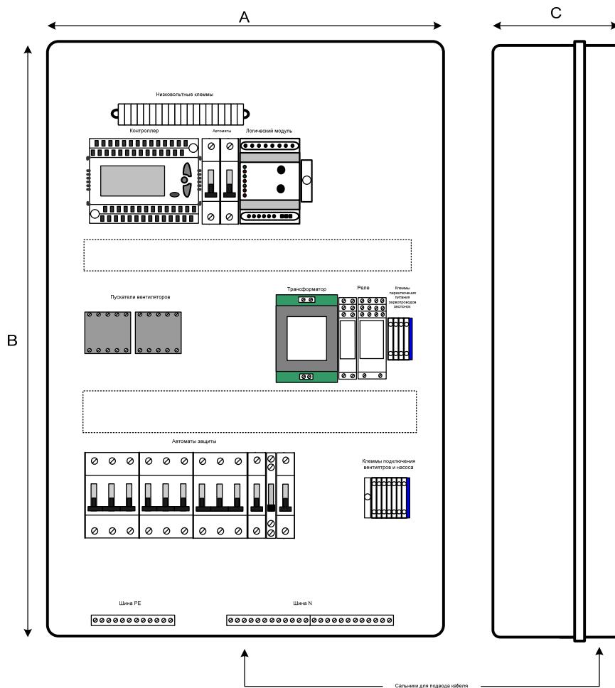
Рисунок 6. Внешний вид блока при открытой крышке.
