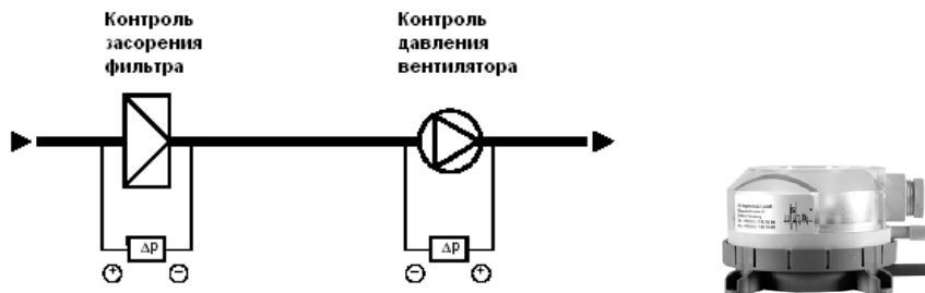
Внешний вид и примеры использования датчиков давления.
