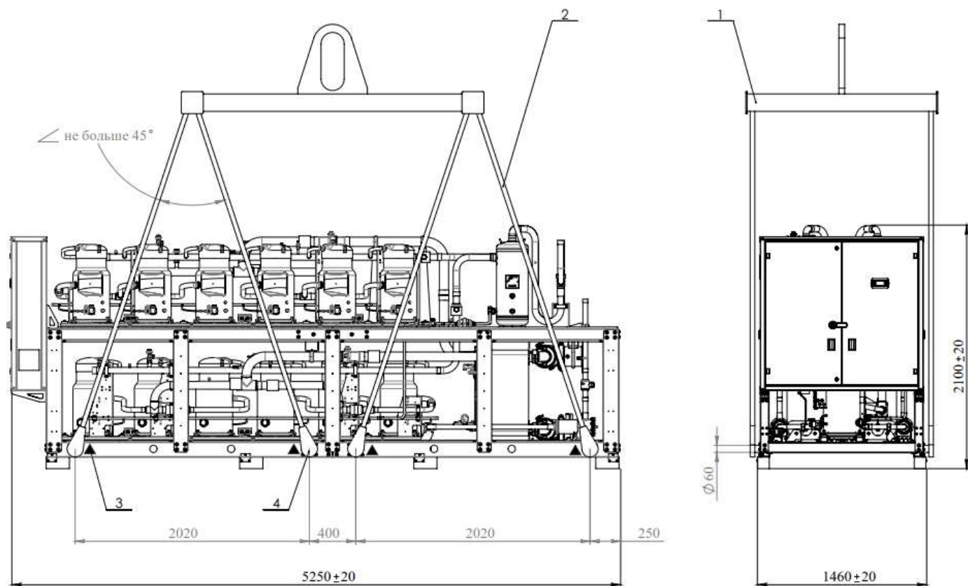
Рис. 4.2.5 Схема строповки чиллера 900
