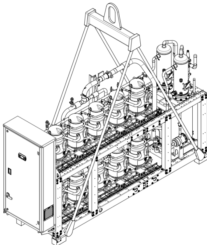
Рис. 4.2.2 Схема строповки чиллеров 500/560
