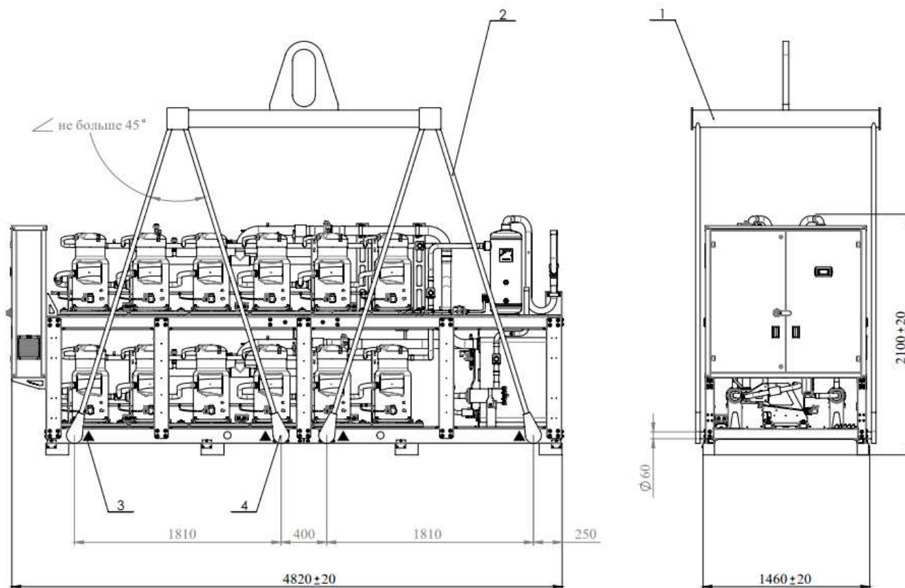
Рис. 4.2.4 Схема строповки чиллеров 720/780
