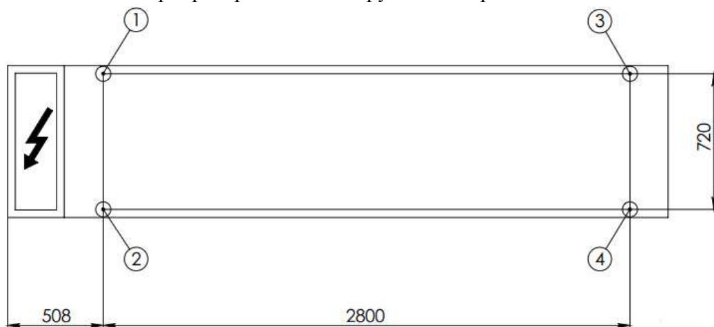
Рис. 4.3.5 Монтаж опор и распределение нагрузки чиллеров 410/460
