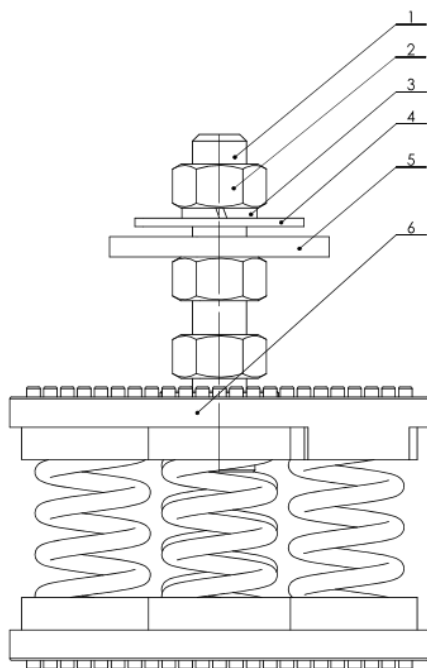
Рис. 4.3.3. Виброопора, способ установки с «домкратом».
