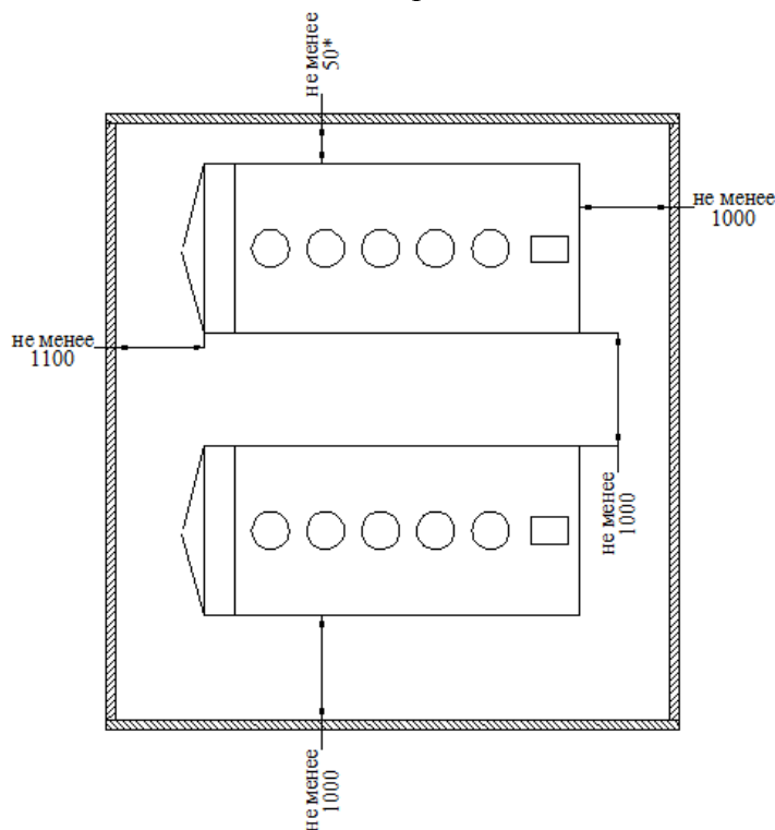
Рис. 4.3.12 Схема установки нескольких чиллеров 410-560*.
