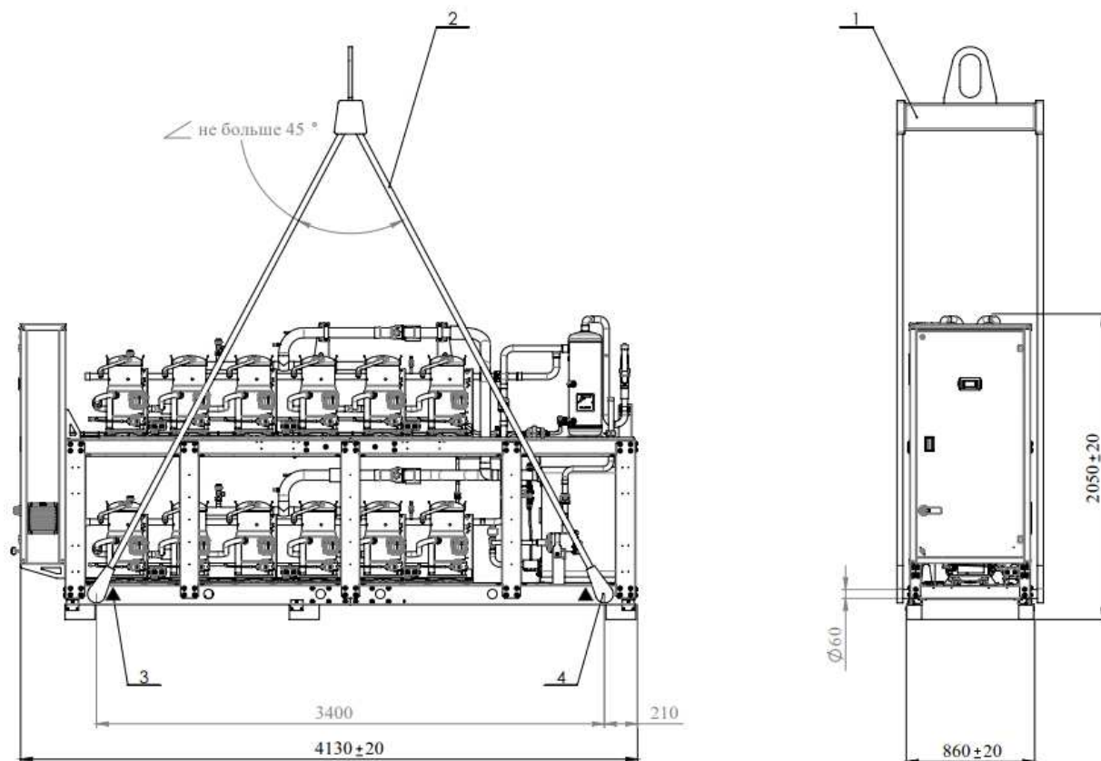
Рис. 4.2.2 Схема строповки чиллеров 500/560
