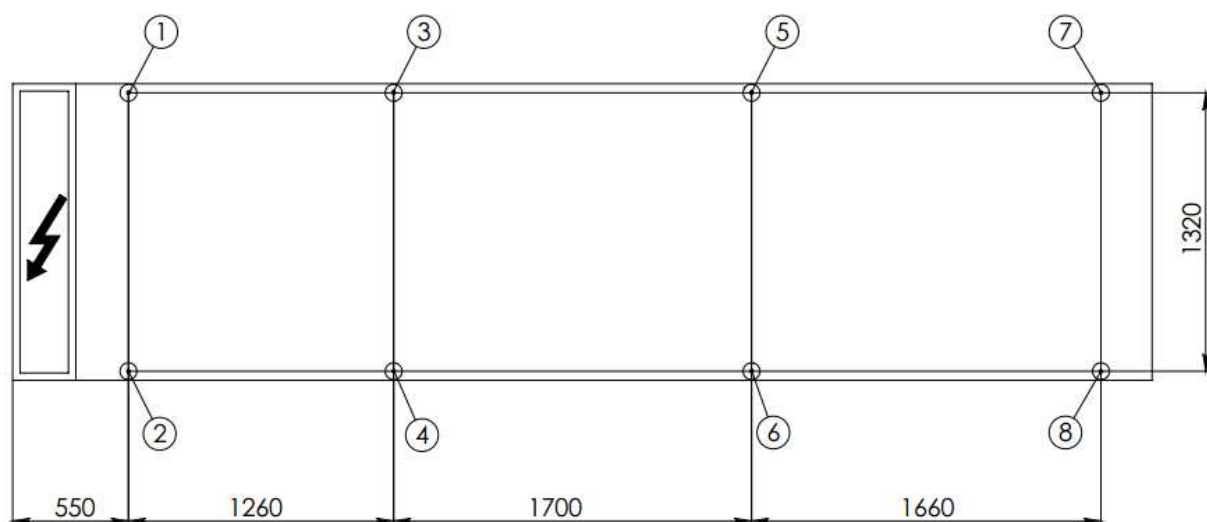
Рис. 4.3.11 Монтаж опор и распределение нагрузки чиллера 1100
