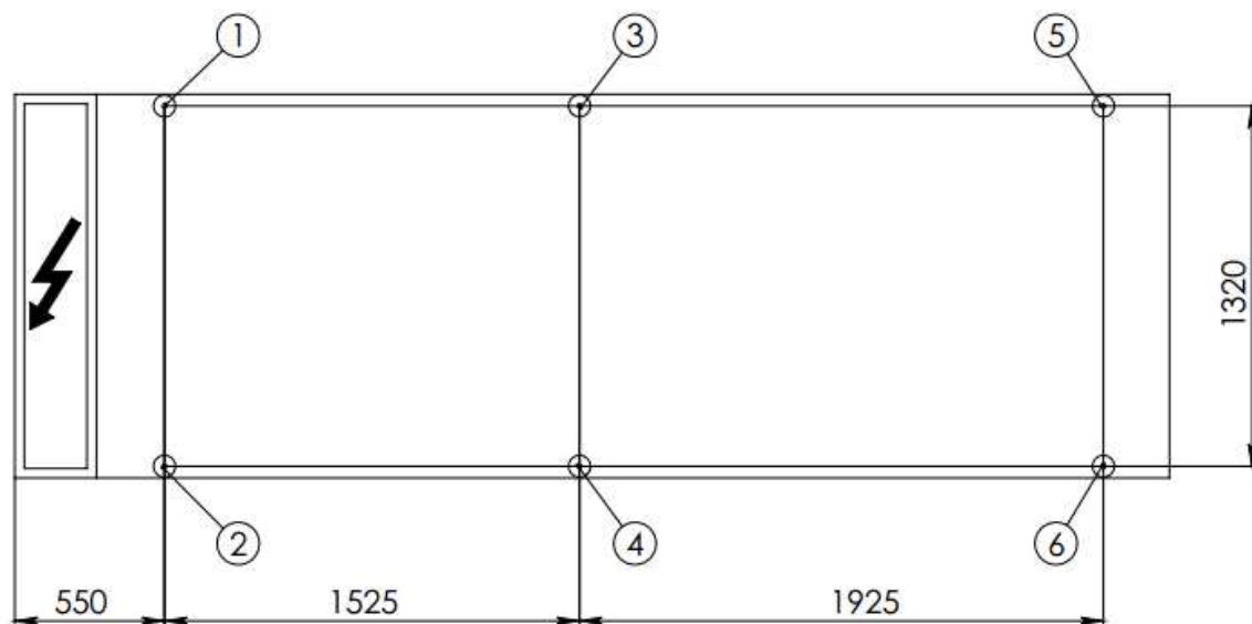
Рис. 4.3.7 Монтаж опор и распределение нагрузки чиллера 630
