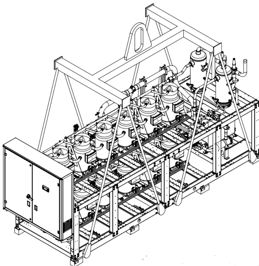
Рис. 4.2.5 Схема строповки чиллера 900
