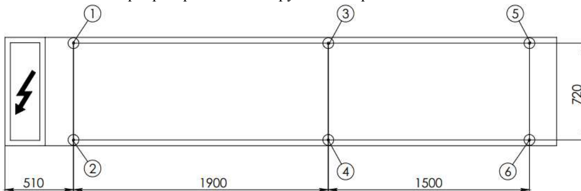
Рис. 4.3.6 Монтаж опор и распределение нагрузки чиллеров 500/560
