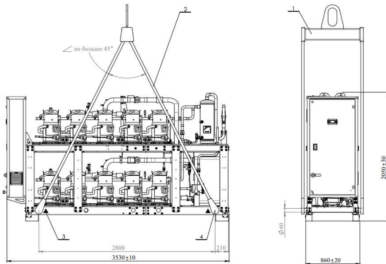
Рис. 4.2.1 Схема строповки чиллеров 410/460
