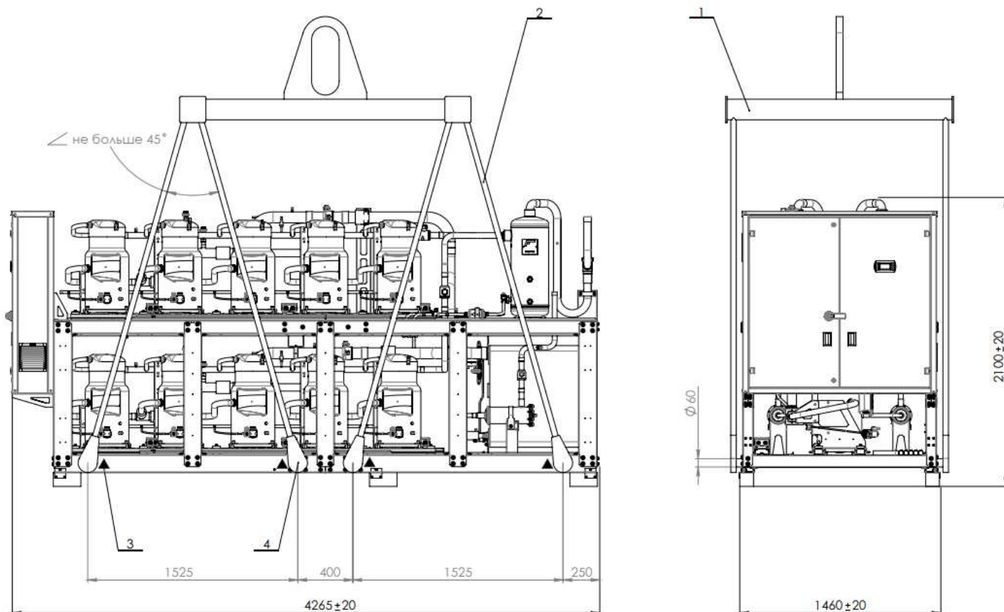
Рис. 4.2.3 Схема строповки чиллера 630
