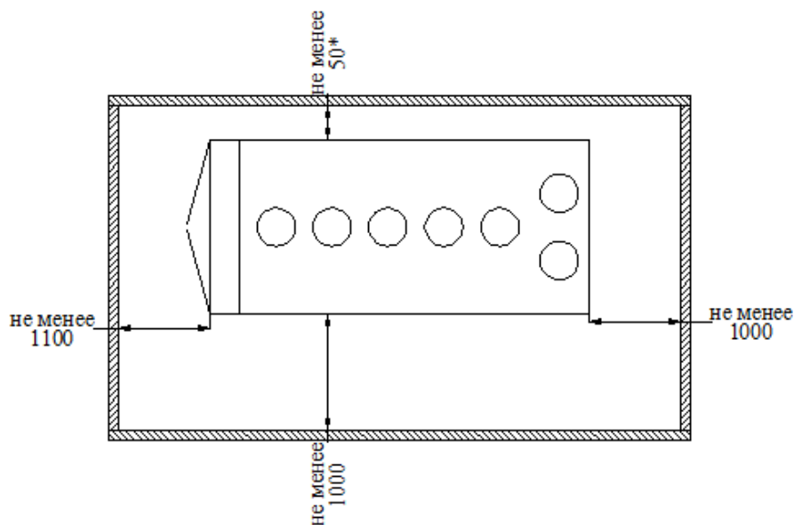
Рис. 4.3.11 Схема установки одиночного чиллера 410-560*.
