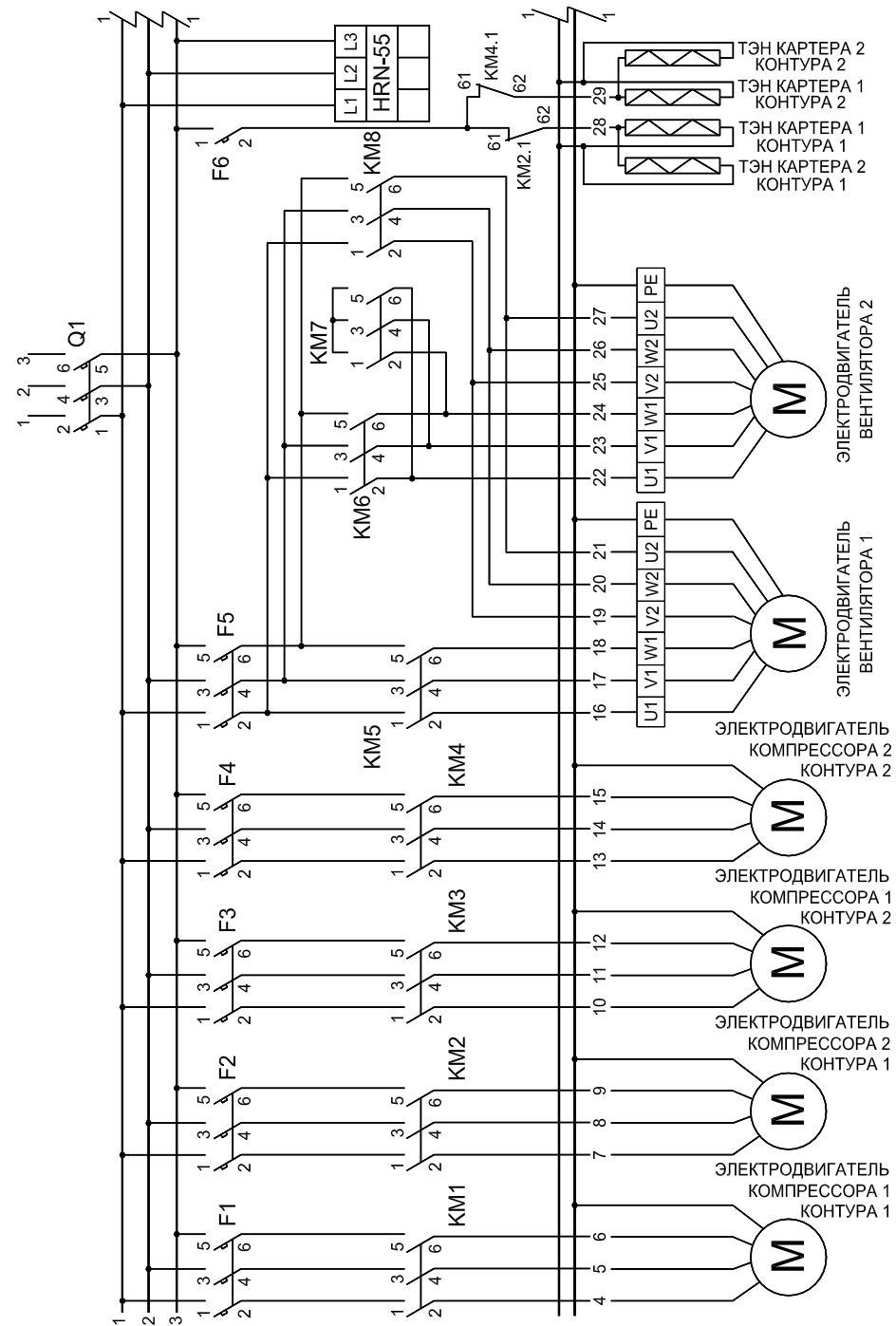
Принципиальная электрическая схема агрегатов (10.С07.03) - модели 080D и 139D (ЛИСТ 1)
